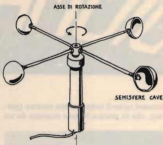
ANEMOMETRO - (VELOCITA')
