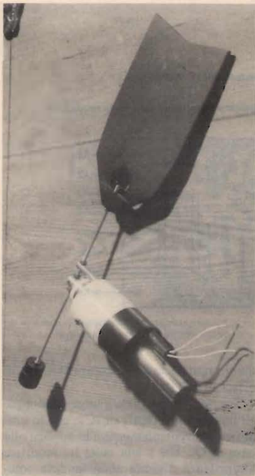
Un prototipo di anemoscopio "Doppia Vela".
