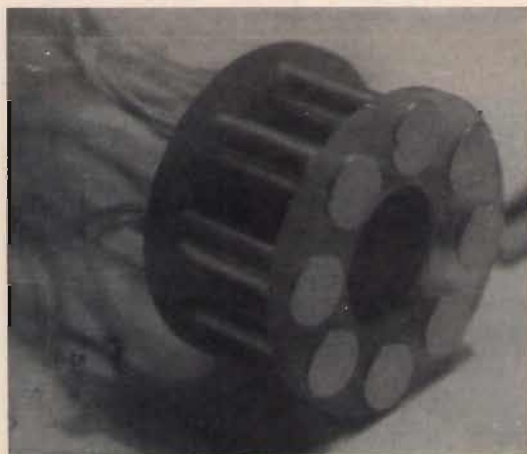
Il "tamburo" degli interruttori reed che andrà posizionato all'interno del contenitore metallico. Sarà tenuto distanziato dal magnete rotante solidale col timone (banderuola) di circa 5 + 6 mm. Il tappo plastico a tenuta del contenitore risulterà interposto appunto tra magneti e interruttori reed.
