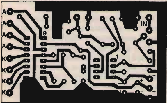
Circuito stampato dell'indicatore di direzione del vento (scala 1:1).
